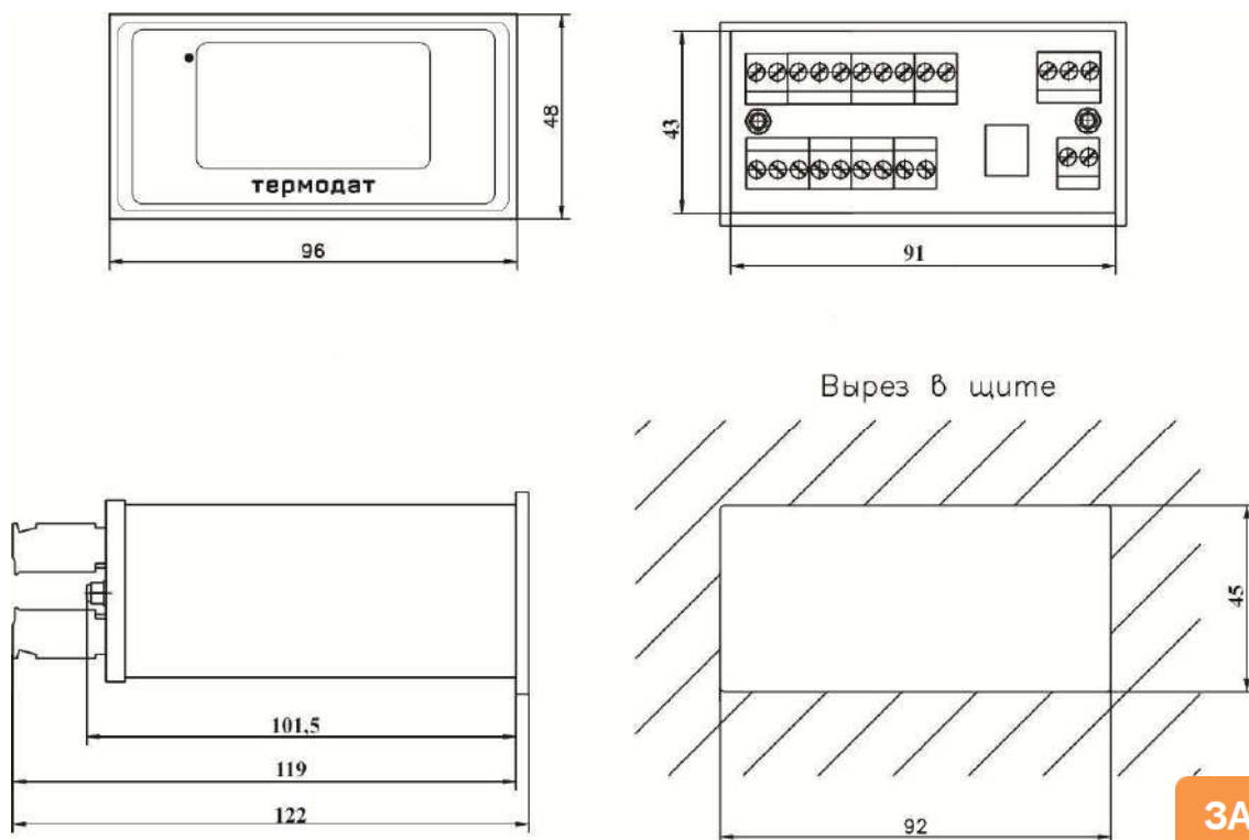
Рисунок 12 – Габаритные размеры прибора Термодат-16М6-Н-(F)-(Eth)
