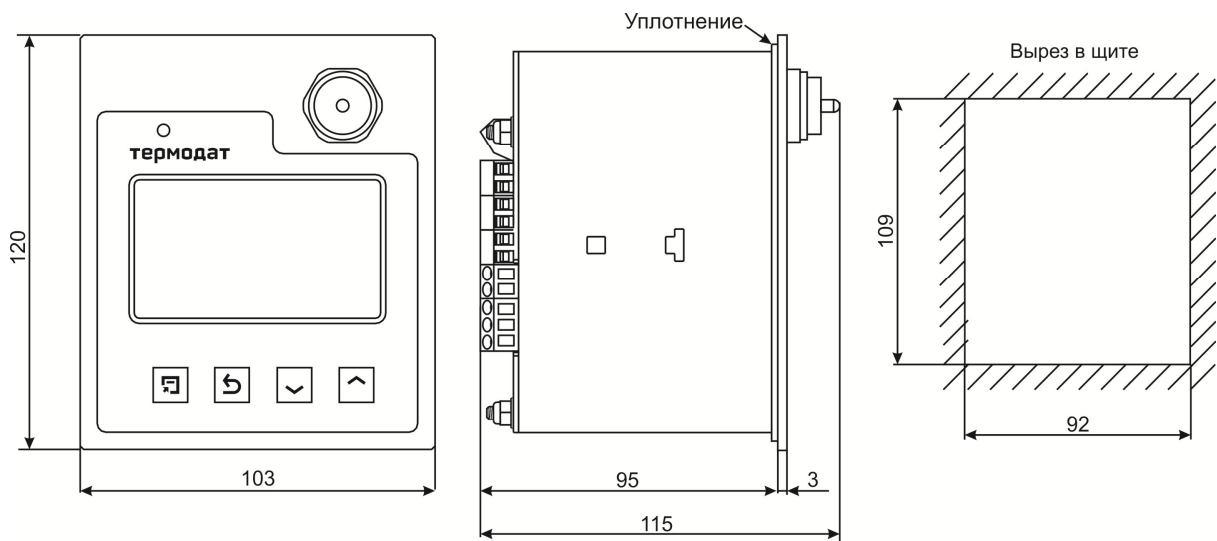
Рисунок 11- Габаритные размеры прибора Термодат-16М6/...../F/IP67пп или Термодат-16М6-А9-(F)
