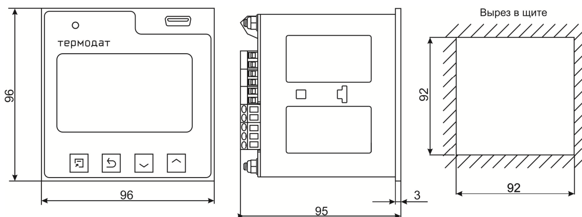
Рисунок 9 – Габаритные размеры прибора Термодат-16М6/...../(F) или Термодат 16М6-А-(F)
