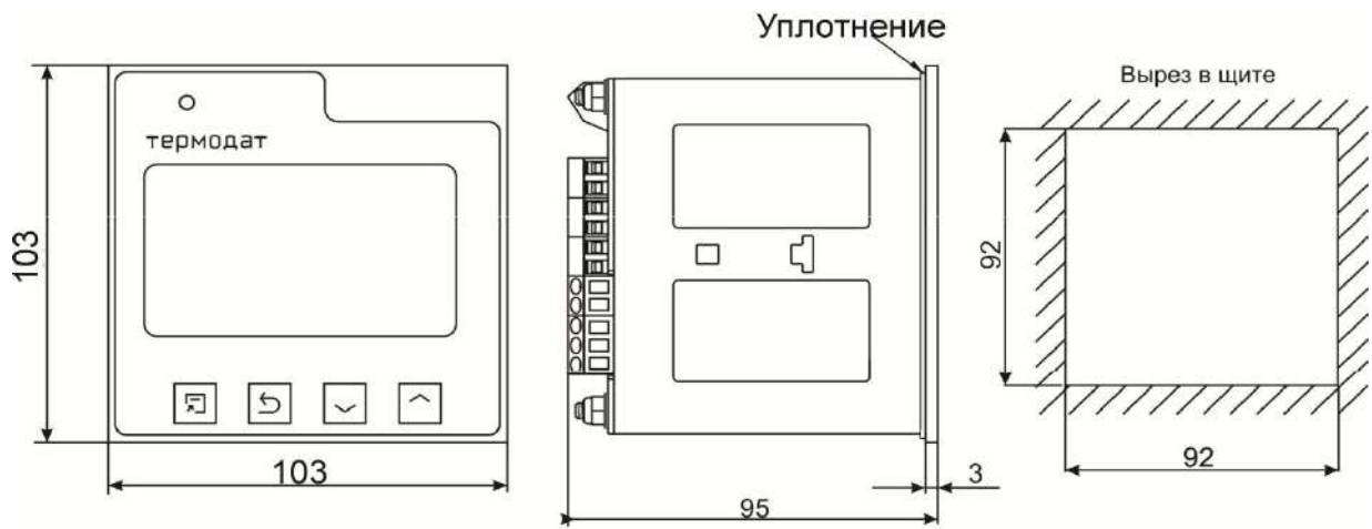
Рисунок 10– Габаритные размеры прибора Термодат-16М6/...../IP67пп или Термодат-16М6-А7
