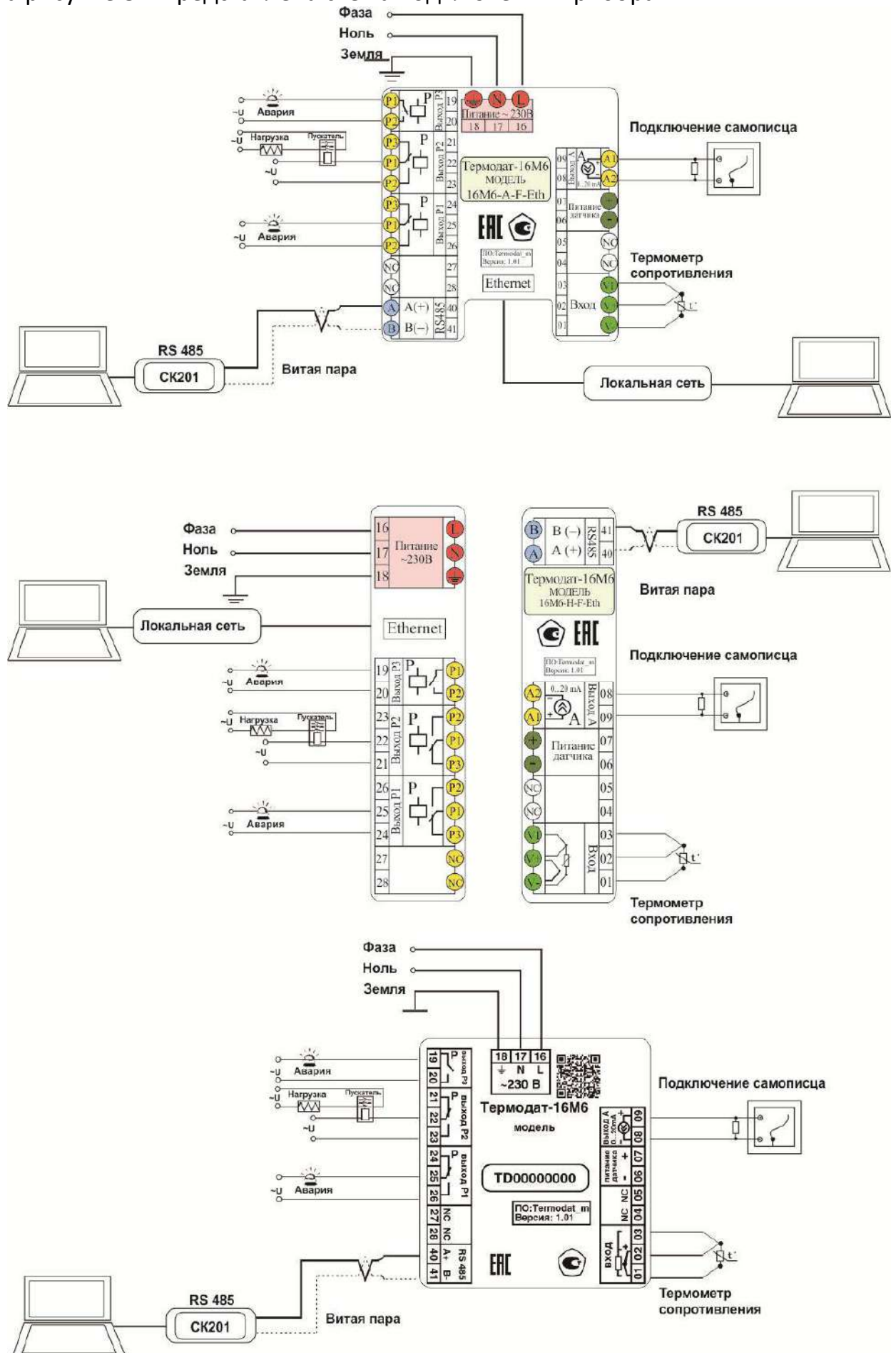
Рисунок 8 - Схема подключения прибора.
