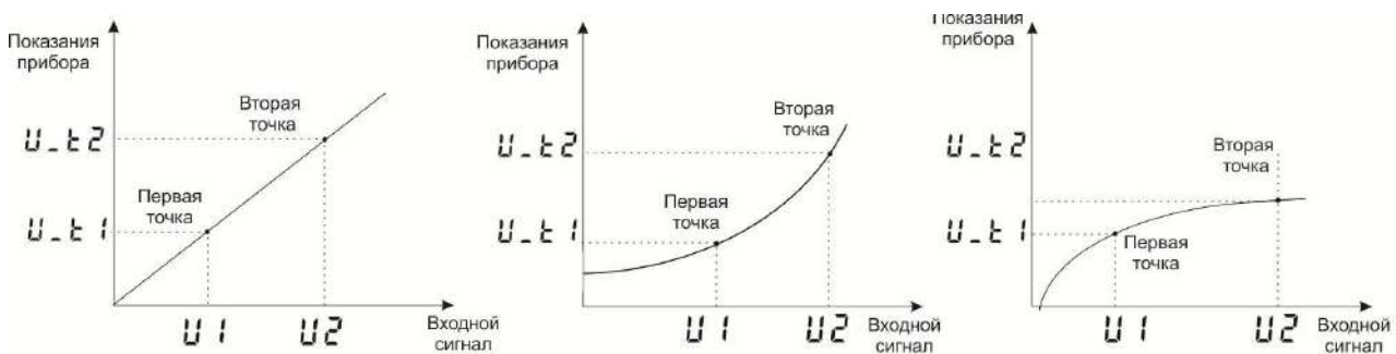
Рисунок 3 – Графики зависимости показаний прибора от входного сигнала при использовании входа типа U.in, PrbL, Sqr и датчика 4-20
