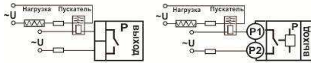
Подключение нагрузки мощностью более 2,3 кВт с помощью электромагнитного пускателя
